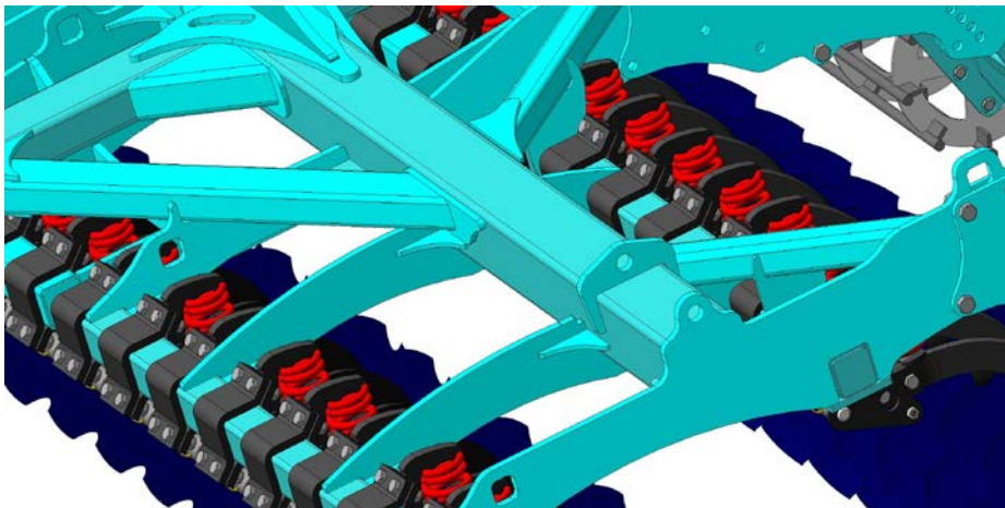
Мощное крепление снуды к раме.
